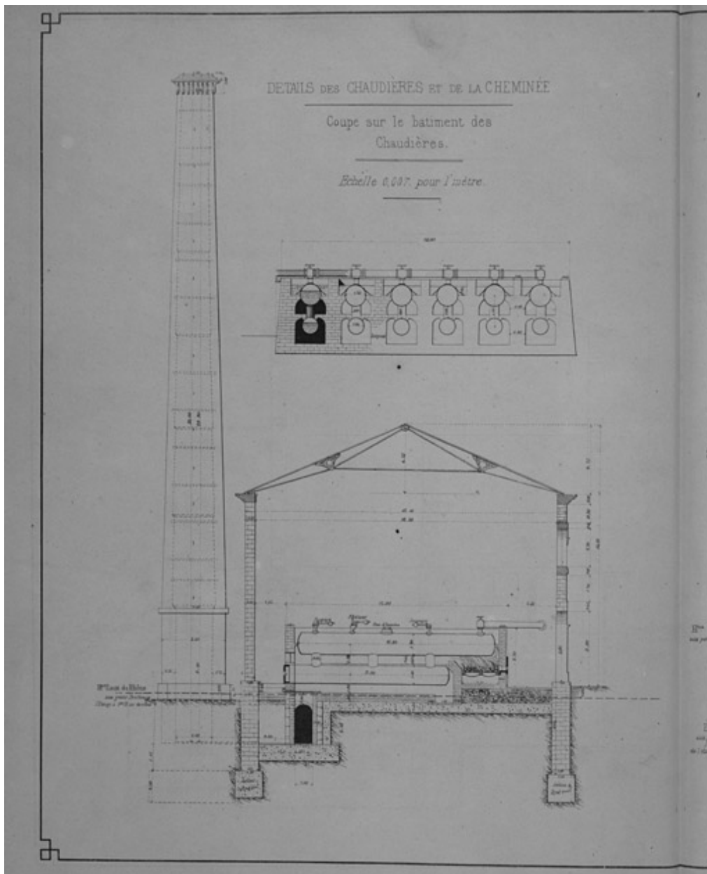
Détail des chaudières et de la cheminée
