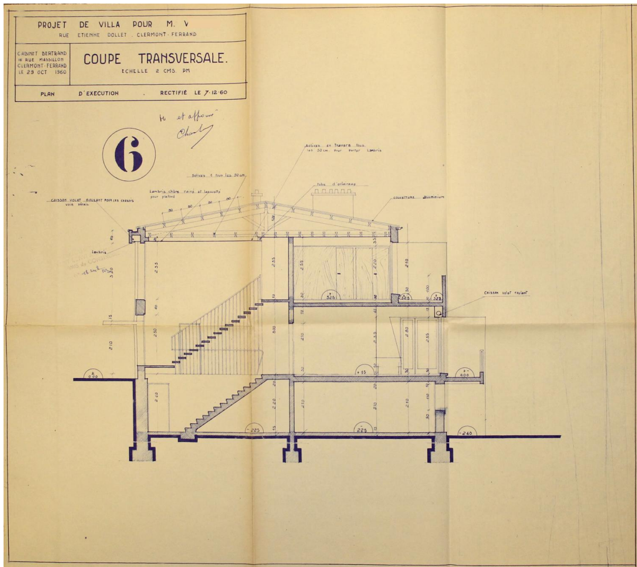
Clermont-Ferrand, la maison V., coupe transversale, Cabinet Bertrand - Jean-Paul Bertrand architecte, octobre 1960 (archives municipales de Clermont-Ferrand).
