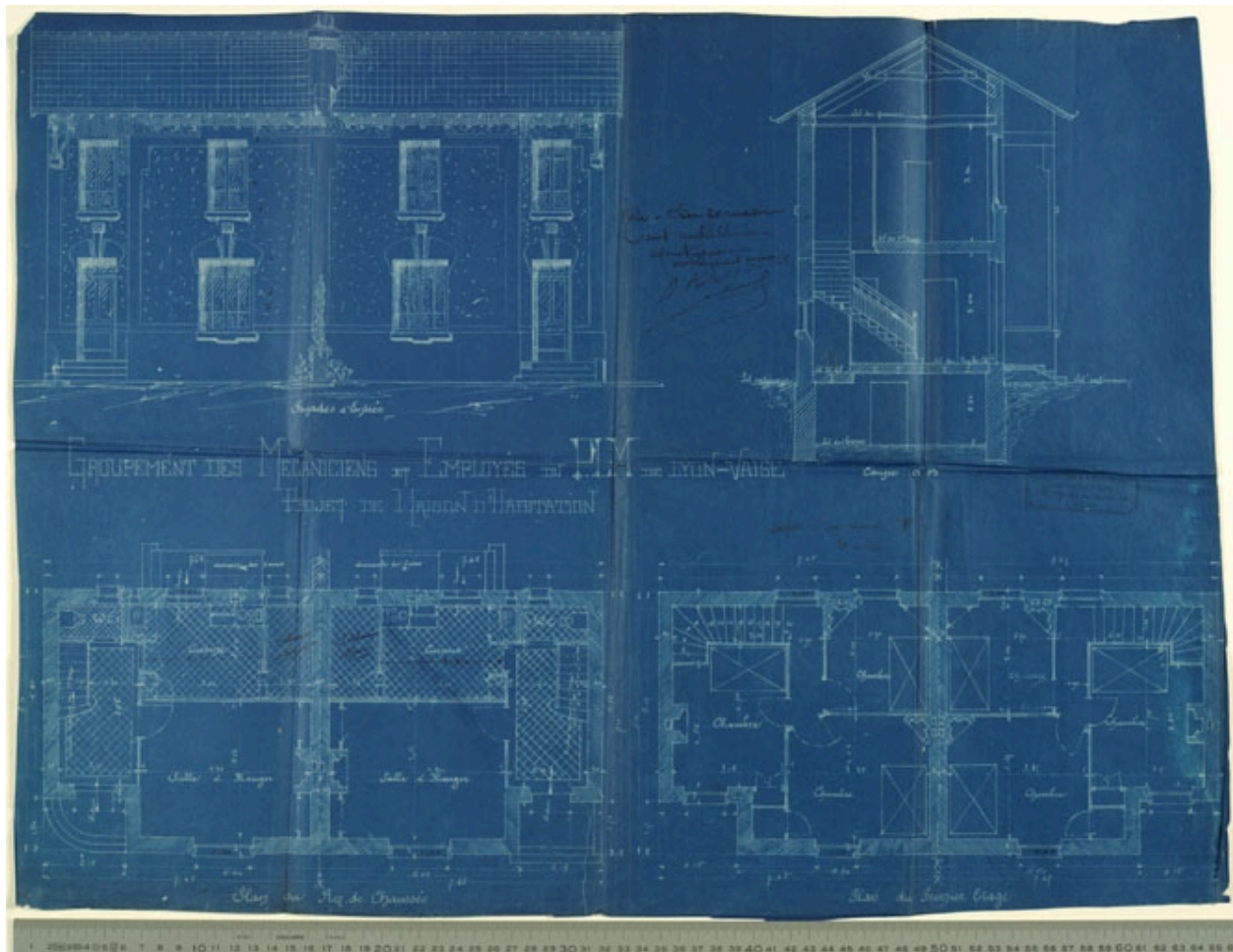
314 WP 58, 1908 permis 629, plans, coupe, façade de maisons jumelles
