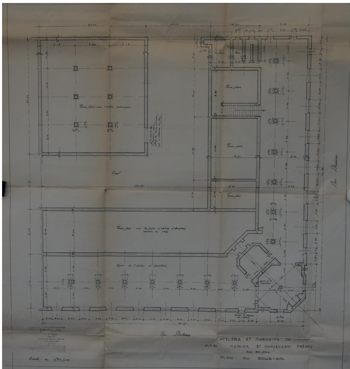
Plan du sous-sol de l'usine Mercier et Chaleyssin 1913 (ACL 314W515-121)
