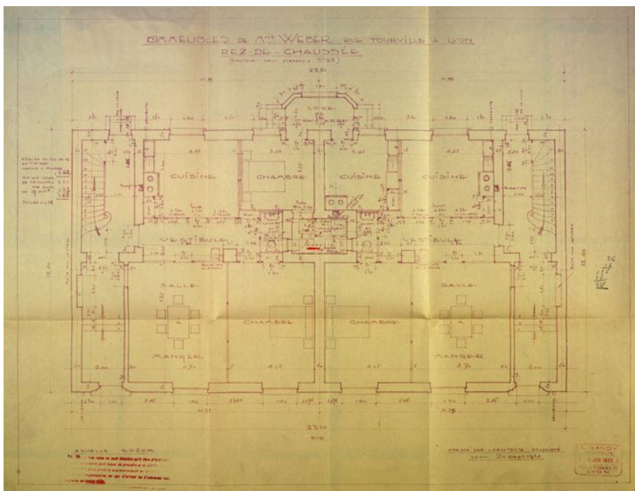
Plan du rez-de-chaussée / L. Gandy architecte, 20 septembre 1934 (AC Lyon. 1097WP 57)
