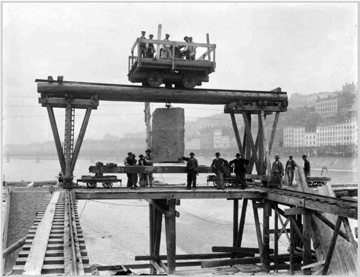
La construction du pont de la Boucle. La pose des maçonneries des piles. [1902]. 1 photogr. : n. et b. (AM Lyon. 15 Ph 1797)
