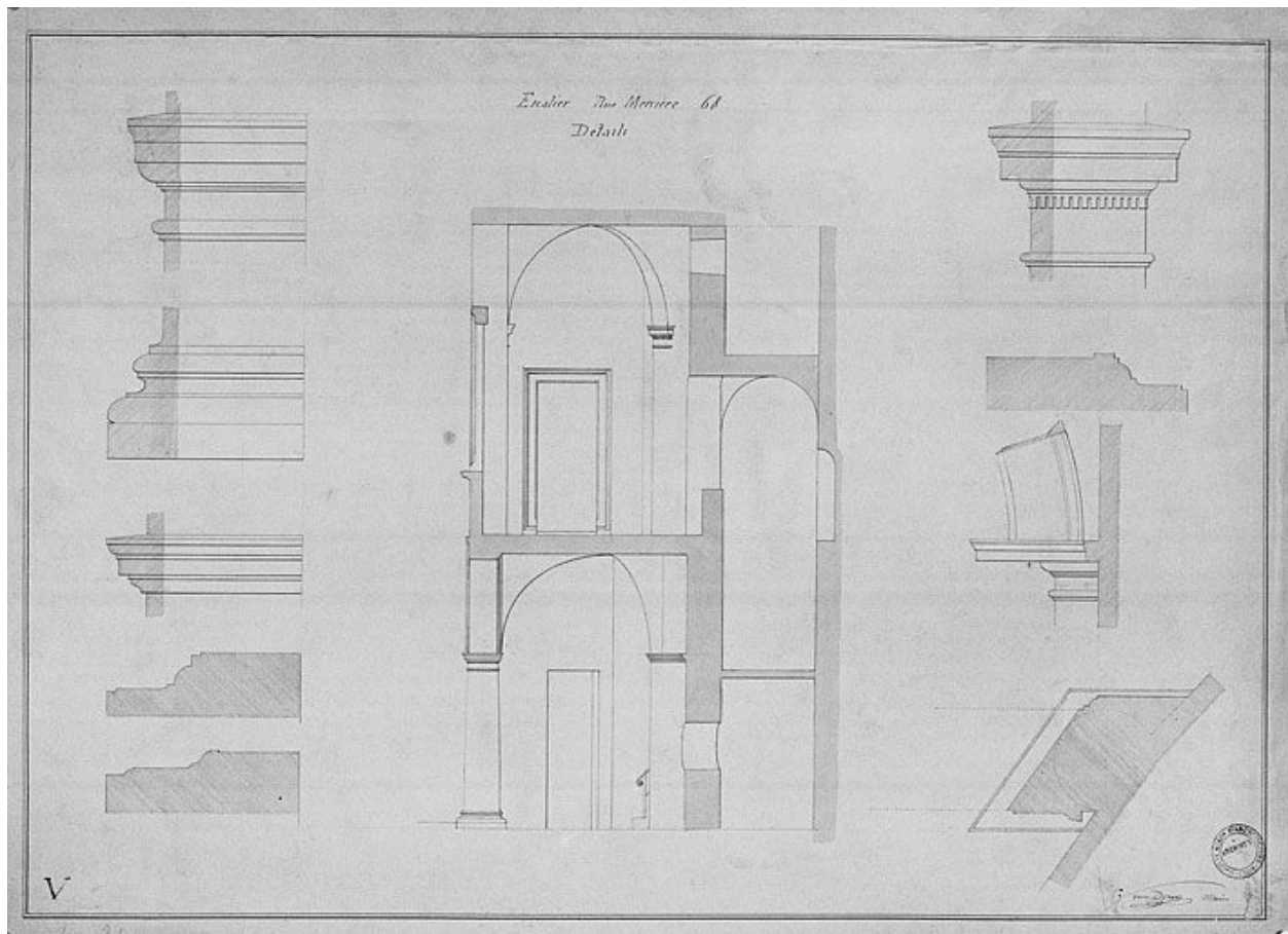
Relevés d'architecture par Marius van Doren. Coupe de l'escalier sur deux niveaux, détails de la modénature
