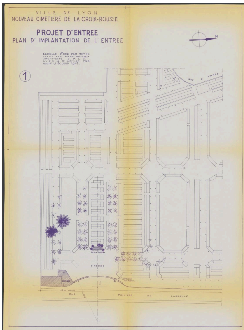
Plan d'implantation de l'entrée, 1, 1968, modifié en 1971
