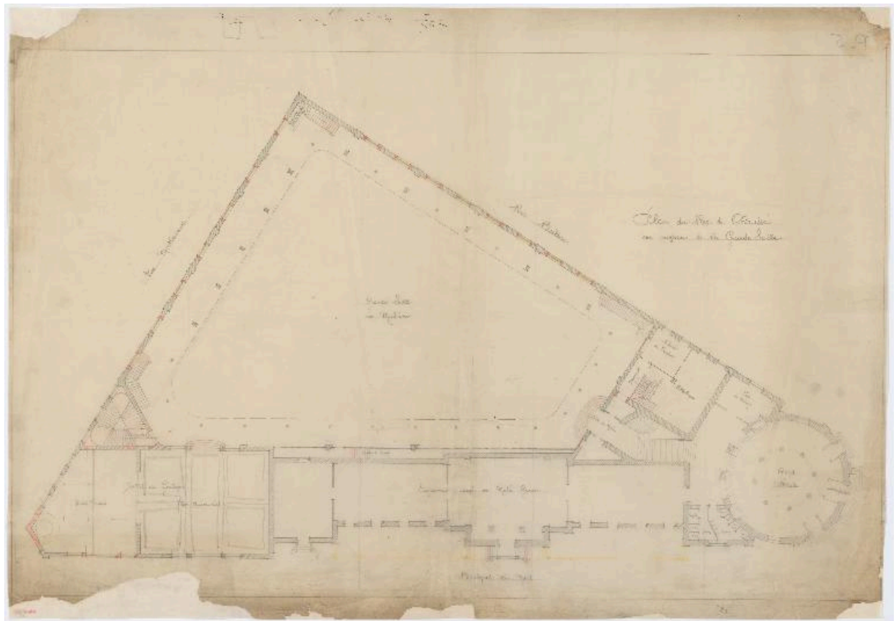
Musée Guimet et Muséum. Plan du rez-de-chaussée au niveau de la grande salle. AC Lyon, 1480 WP 225 M
