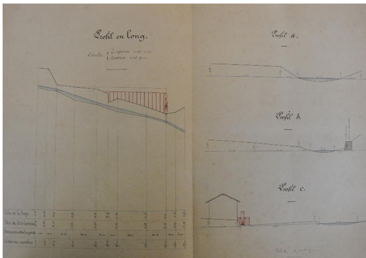
Plan de la scierie, 1889 (FR.AD073, 82S15).
