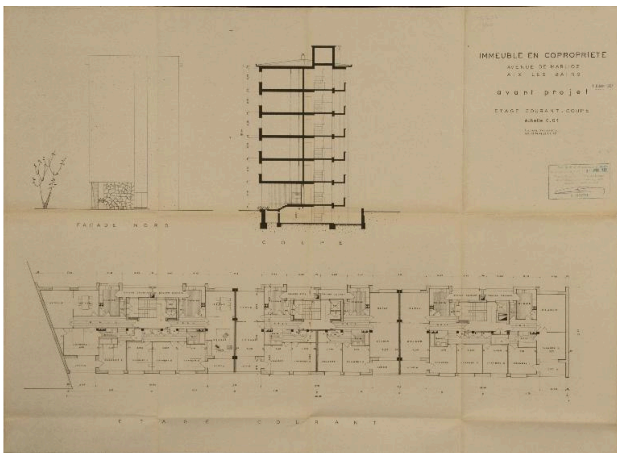
Etage courant et coupe, 1957
