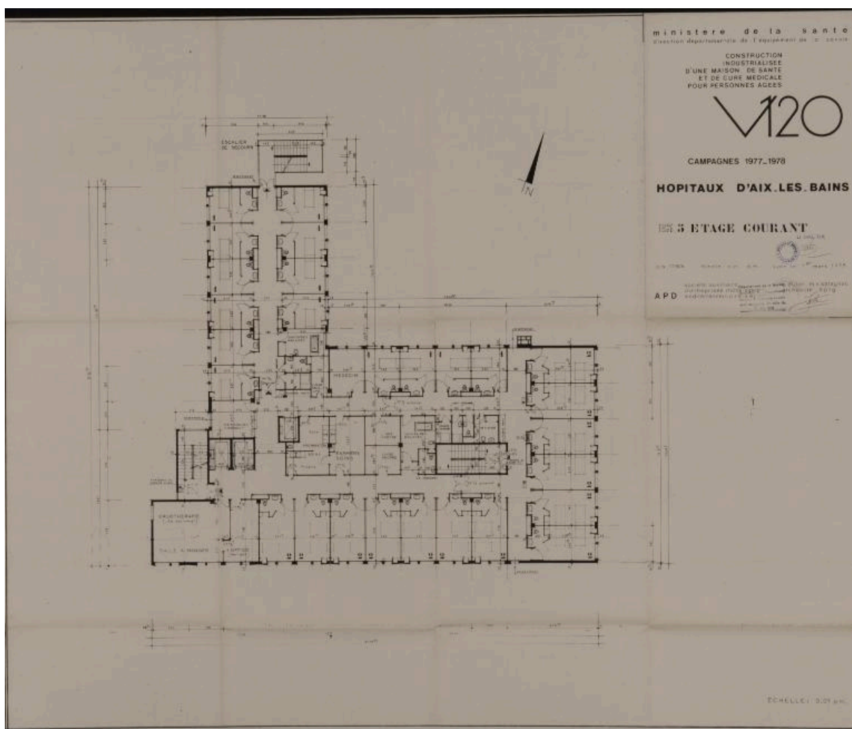
Plan de l'étage courant
