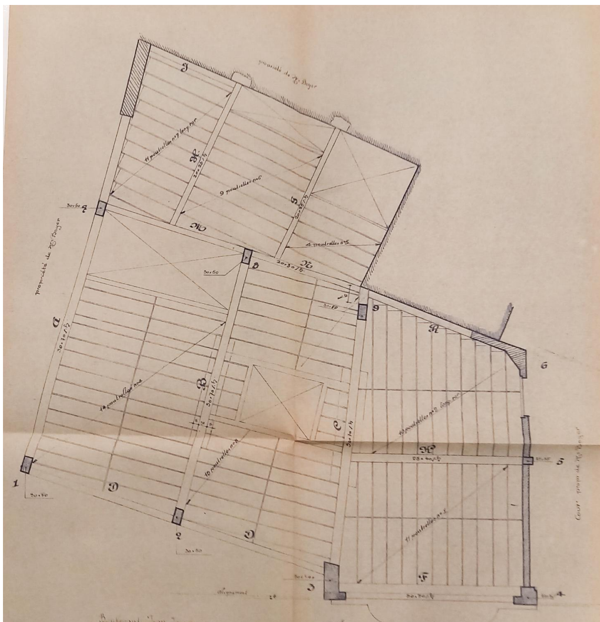
Plan des toitures, implantation du bâtiment (agrandissement 1941)
