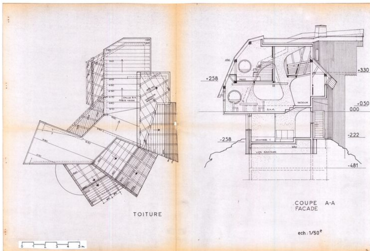
Projet de 1979. Plan de toiture. Coupe A-A, façade / J. Labro (A. privées J. Labro)
