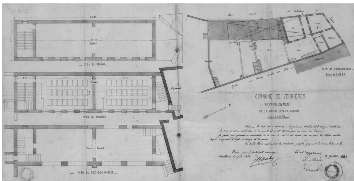
Commune de Verrières. Agrandissement de la maison d'école - garçons. 1883. Plan à l'encre et lavis sur toile huilée, 1883 AC Verrières-en-Forez. Chemise 1883. Agrandissement école de garçons. Jean-Baptiste Dulac.
