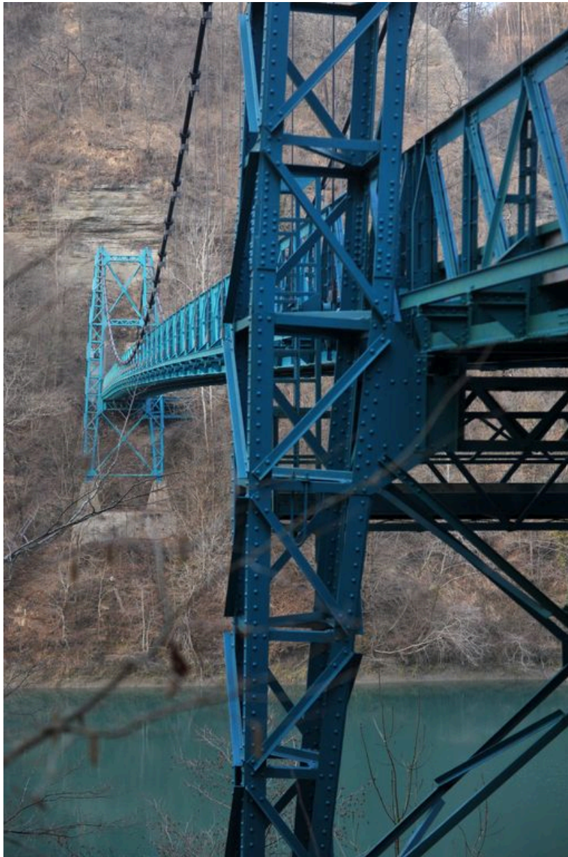
Pylône gauche, vue de détail : structure métallique ; travée centrale et pylône droit en arrière-plan (depuis la rive gauche)
