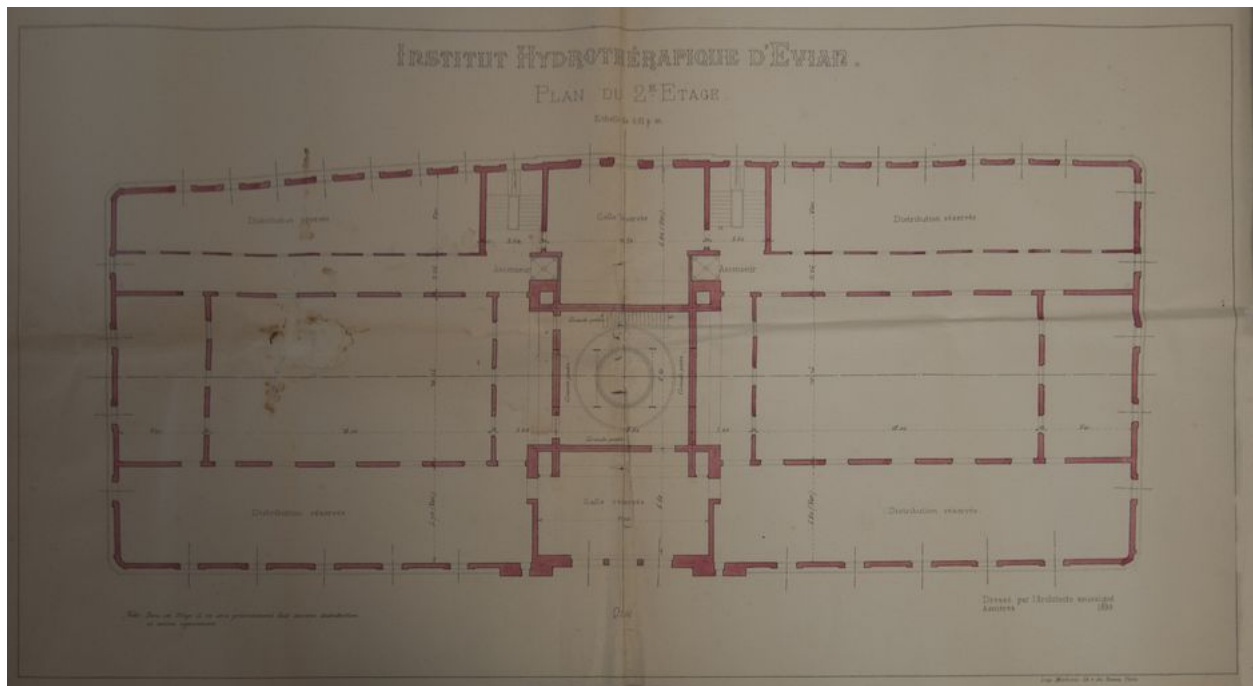
Institut Hydrothérapique d'Évian. Plan du 2ème Etage, novembre 1899. Plan. Archives départementales de la Haute-Savoie © Archives départementales de la Haute-Savoie. 2 O 946
