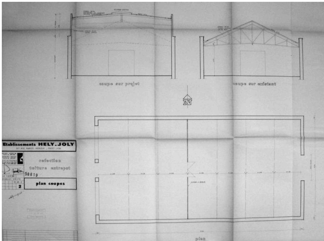
Plans et coupes, Réfectoire toiture et entrapôt, 247 rue Marcel Mérieux, 1 juin 1981 par René Genin et Gérard Favier architectes, échelle 1/50. (Arch. mun. Lyon)
