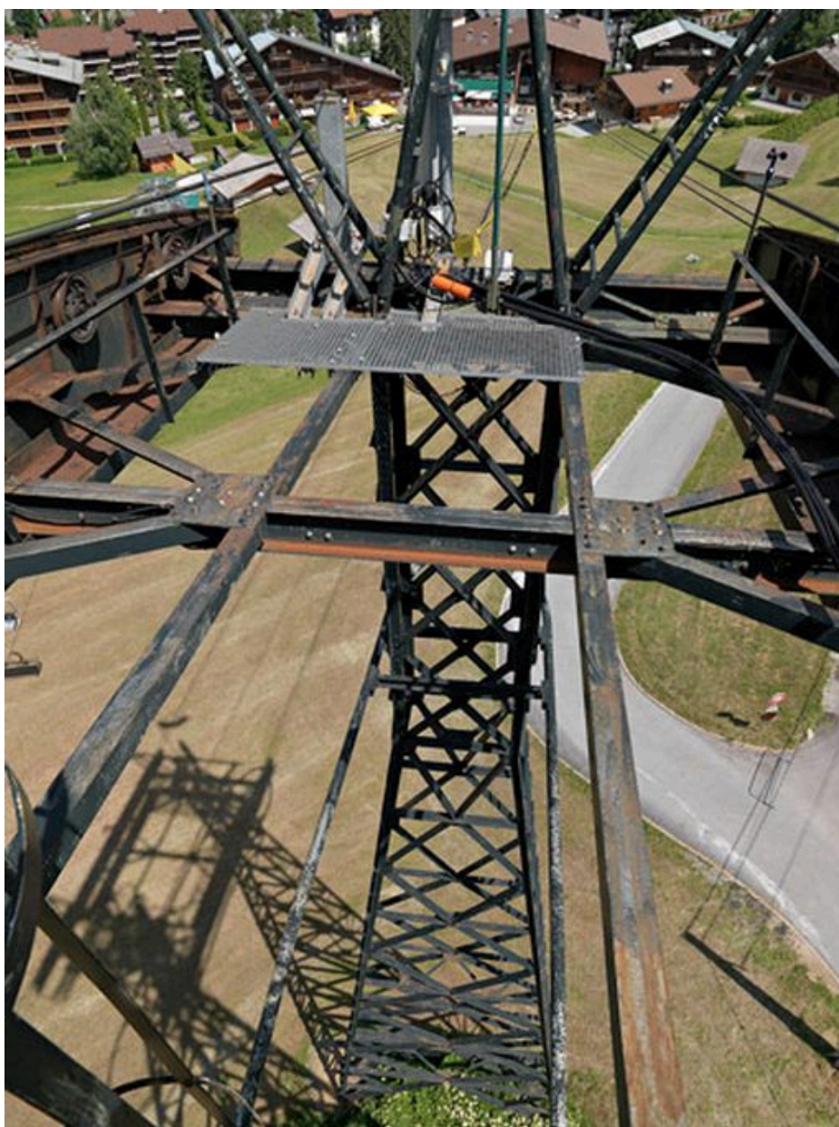
Détail de l'accrochage des câbles de montée et de descente de part et d'autre du pylône
