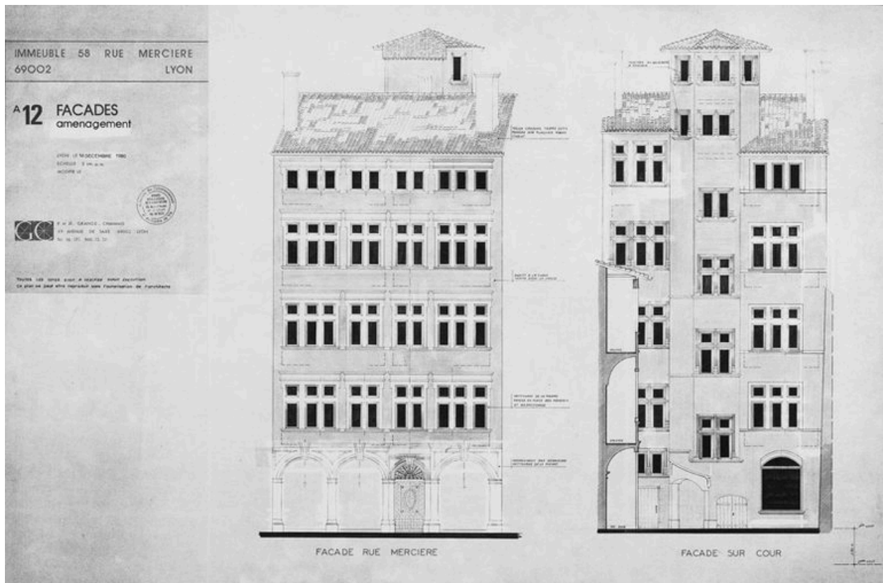
Elévations rue Mercière et sur cour : projet d'aménagement. 1980 CRMH Rhône-Alpes. 1 I 11 MHAA-99-463
