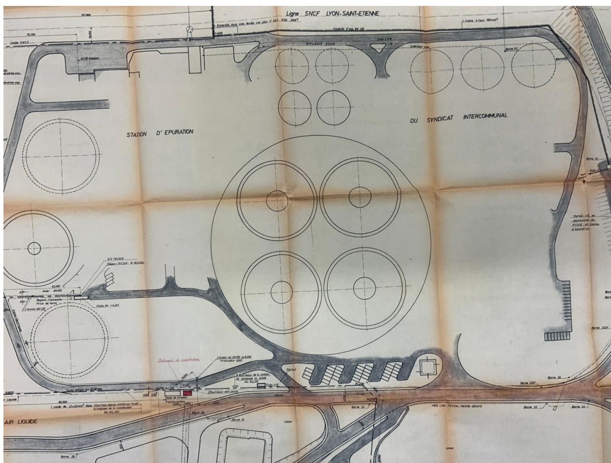
Plan de la station d'épuration, 1976 (AC Pierre-Bénite : 203 – 68)
