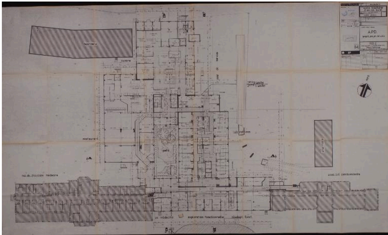
Plan du rez-de-jardin
