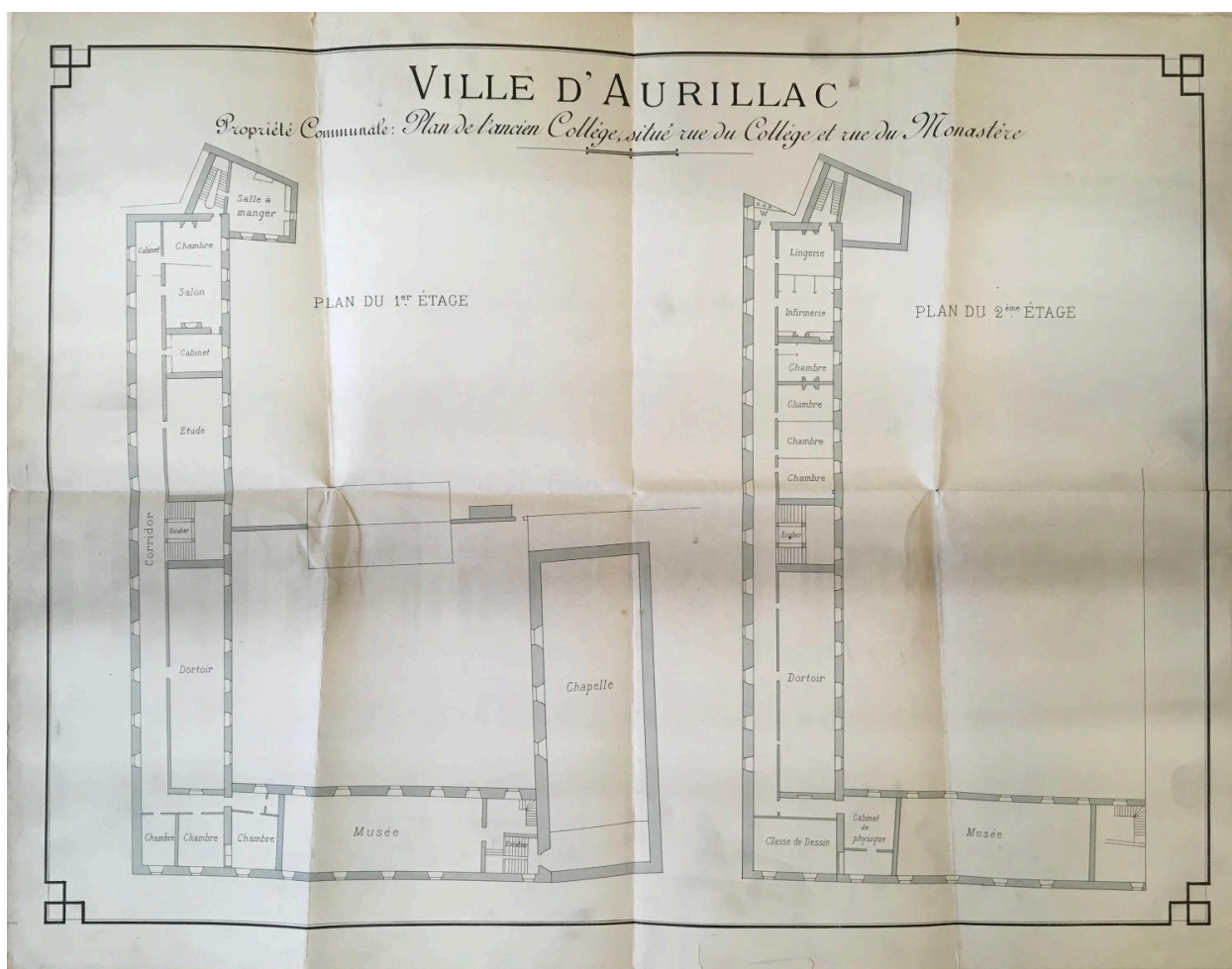
Plan des 1er et 2e étages par L. Courbaize, 1893 (AD Cantal, E DEP 1500/1487)
