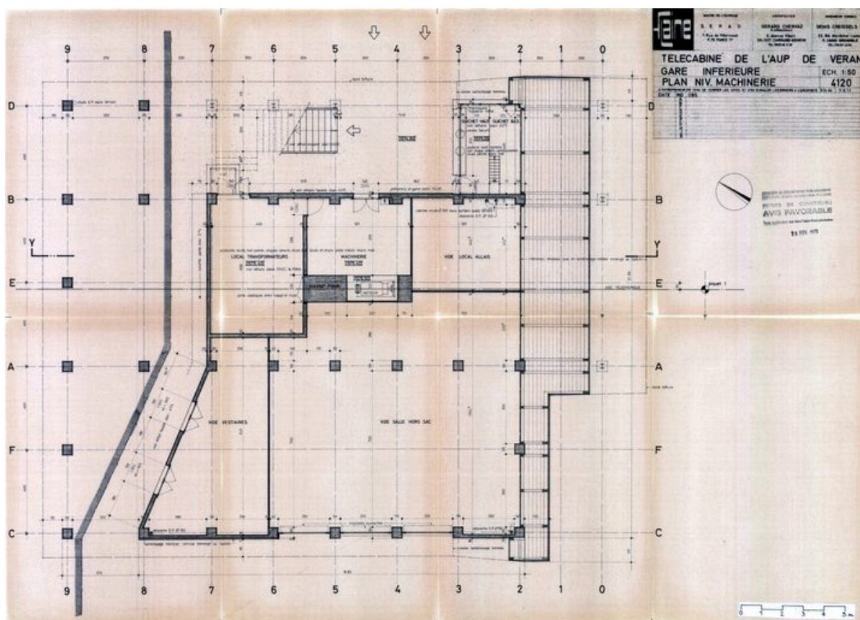
Plan niveau machinerie. Gérard Chervaz architecte, Denis Creissels ingénieur conseil, 11 août 1972 (AC Magland)
