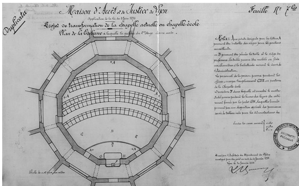
Transformation de la maison d'arrêt et de justice de Lyon en prison cellulaire : chapelle-école, plan de la tribune, H. Moncorger, 1885. calque entoilé, 10 janvier 1885, 26,5 x 44 AD, Rhône. 1 Y 283
