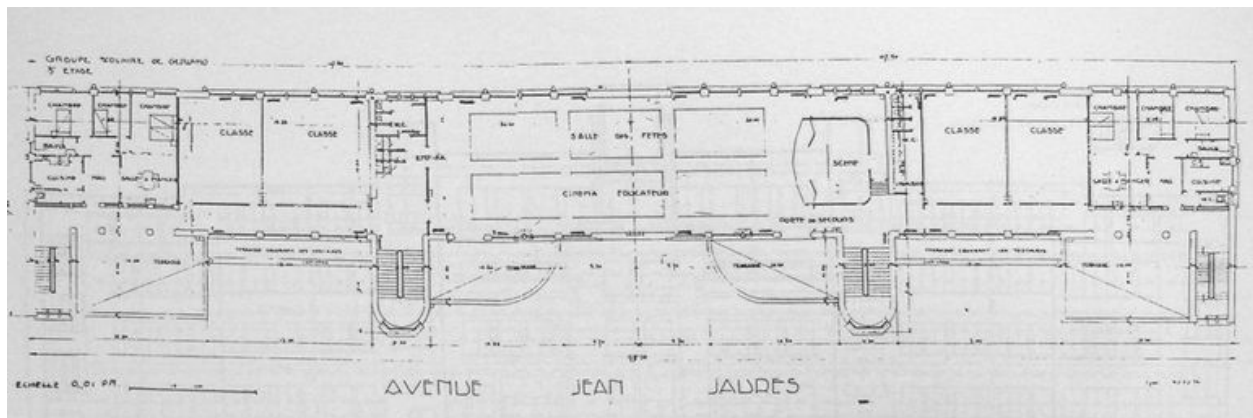
Plan du 3e étage, Réalisation Ecole primaire de Gerland, 3 mars 1932 par V.-A. Robert et A.-E. Chollat architectes, échelle 1/100. (AC Lyon)
