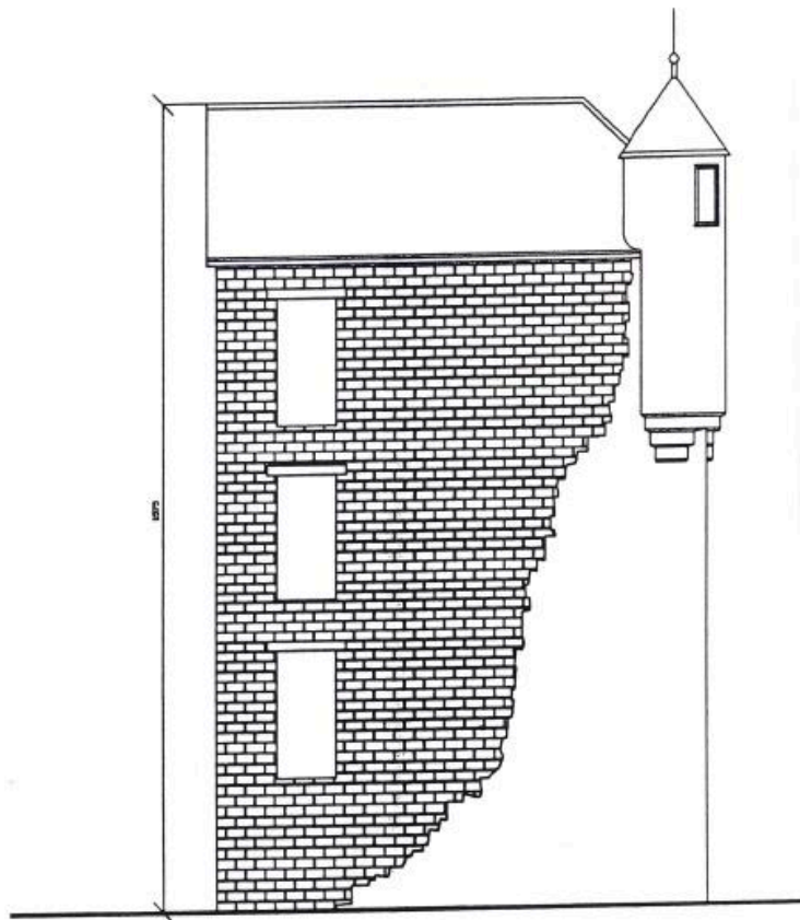
ÉTAT DES LIEUX ACADE NORD ECH:1/100
