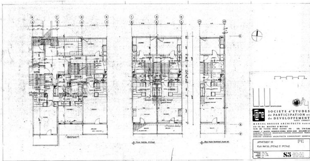
Plan partiel des 2e et 3e étages. Marcel Breuer architecte, 1er juillet 1976 (AC Arâches-la-Frasse)
