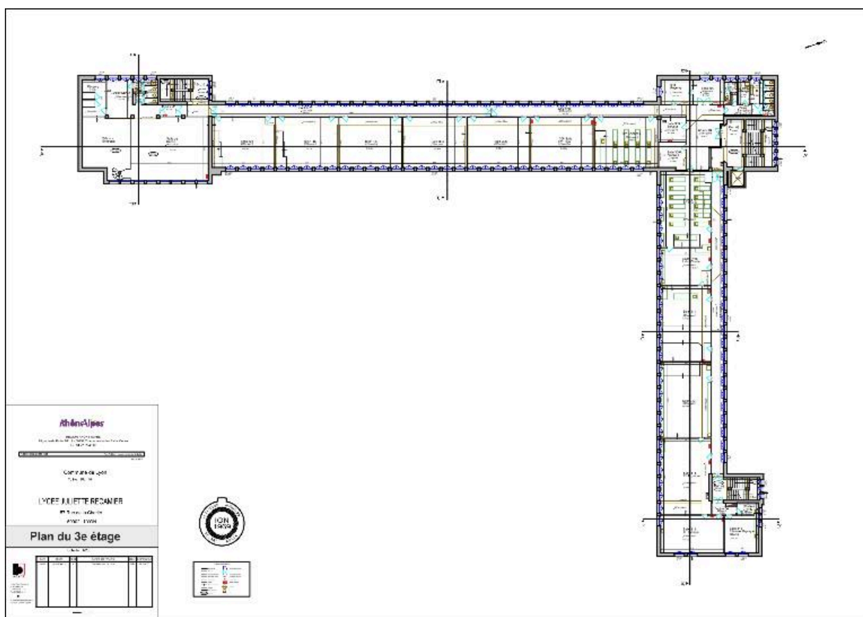
Plan du 3e étage. Dess. AGATE, 2012
