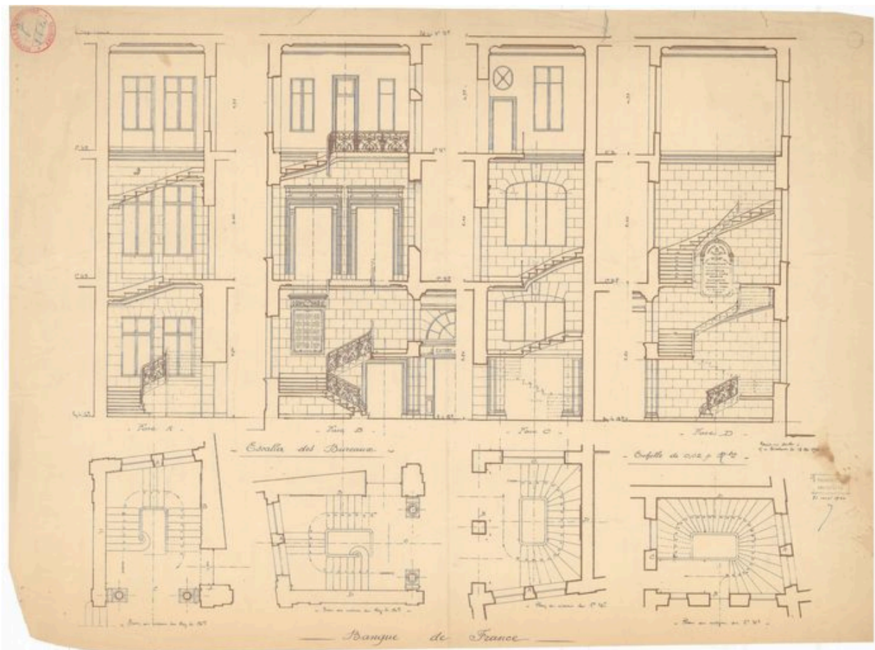
Plans et coupes du nouvel escalier (1920) menant à l'étage des bureaux (premier étage) (Banque de France, service du Patrimoine Historique et Artistique, non coté, dessin de Xavier Thoubillon).
