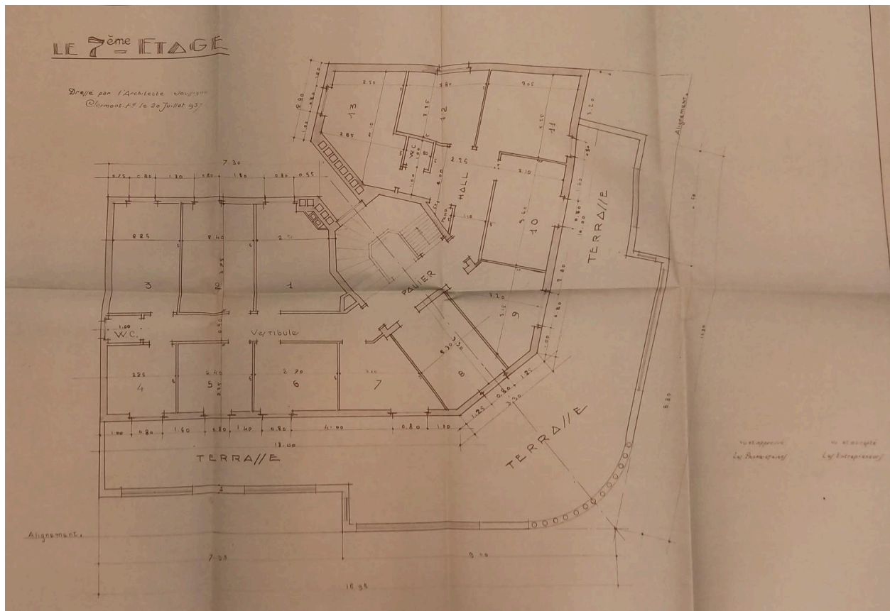
Plan du septième étage. Comparaison n°76 bd Cote-Blatin (projet non réalisé)
