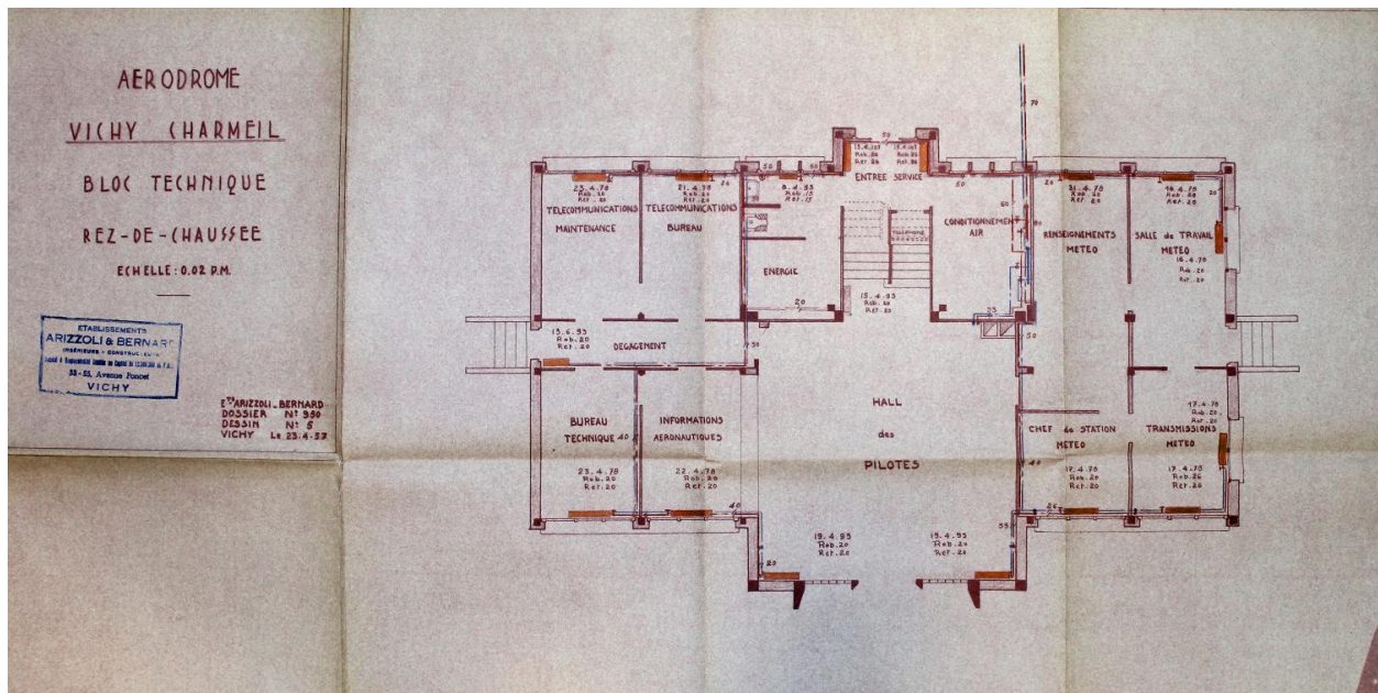
Plan du rez-de-chaussée du bloc technique de l'aérogare de Vichy-Charmeil, 1957, Service technique des bases aériennes (Archives municipales de Vichy).
