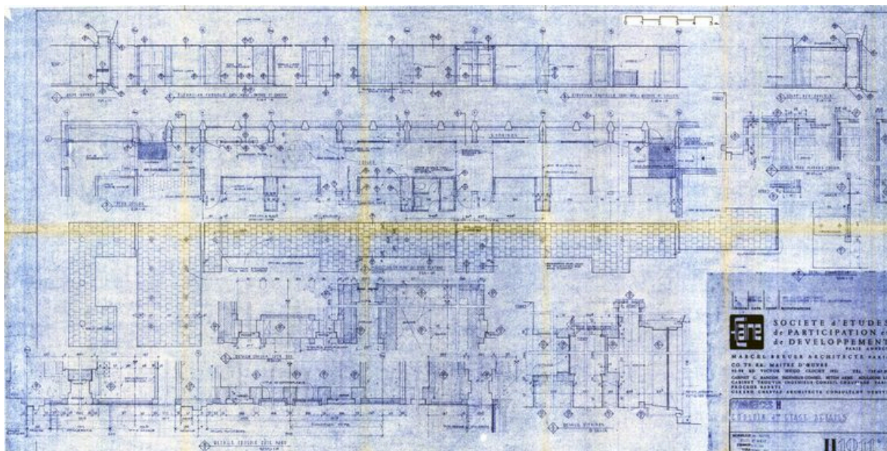
Commerces H. Couloir du 1er étage. Plan et élévations. Détails. Marcel Breuer architecte, 29 novembre 1967 (AC Arâches-la-Frasse)
