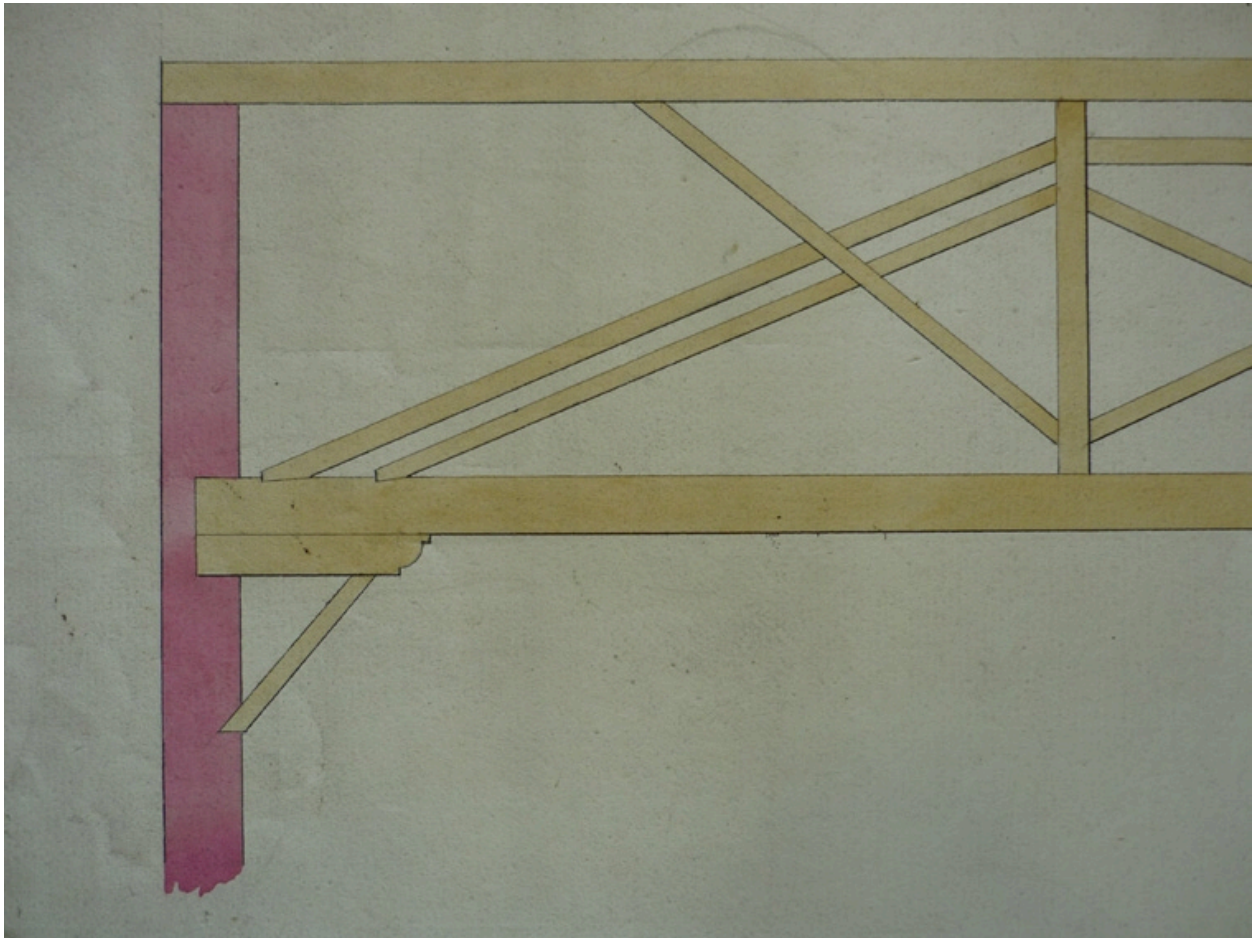
Elévation d'une charpente, s.d. (détail de la partie gauche). Plan AC Lyon. Fonds des HCL ; 2OP686
