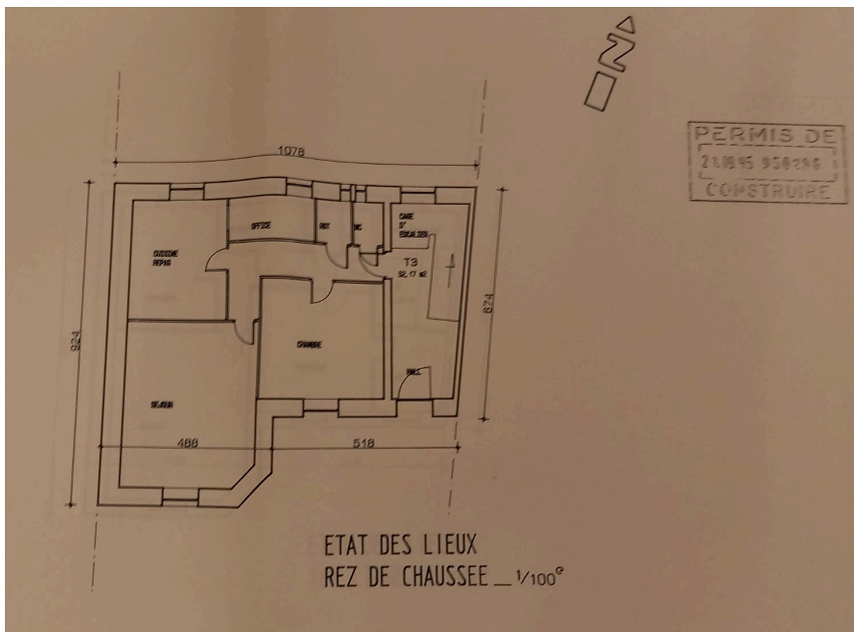
Plan du rez-de-chaussée, état des lieux avant transformation (1995)
