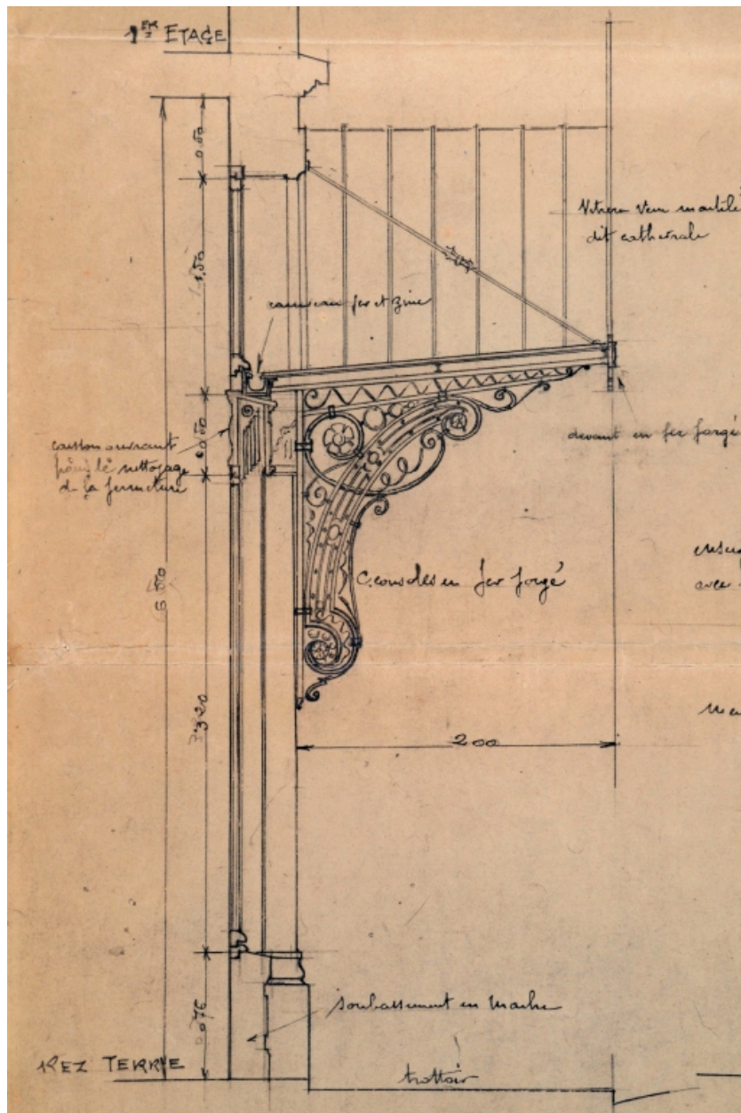
Profil d'une console de la marquise
