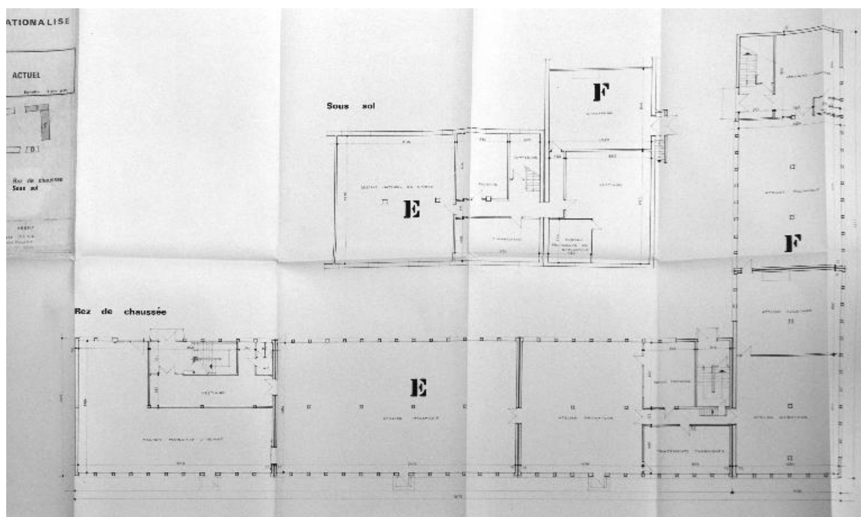
Lycée Technique Nationalisé, Plan bâtiments E et F sous-sol et rez-de-chaussée, A. Profit Mai 1974 (AC Ugine, 6 W 106)
