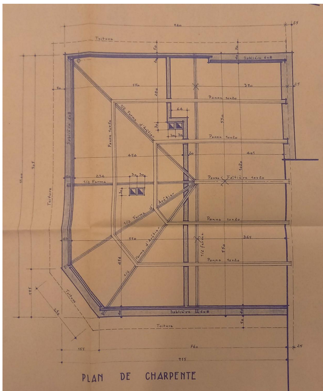
Plan de la toiture
