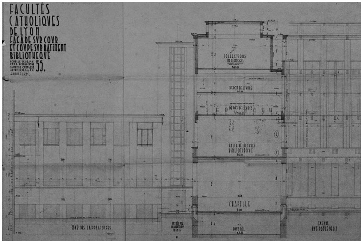
Façade sur cour et coupe du bâtiment de la bibliothèque, Georges Curtelin, 1938
