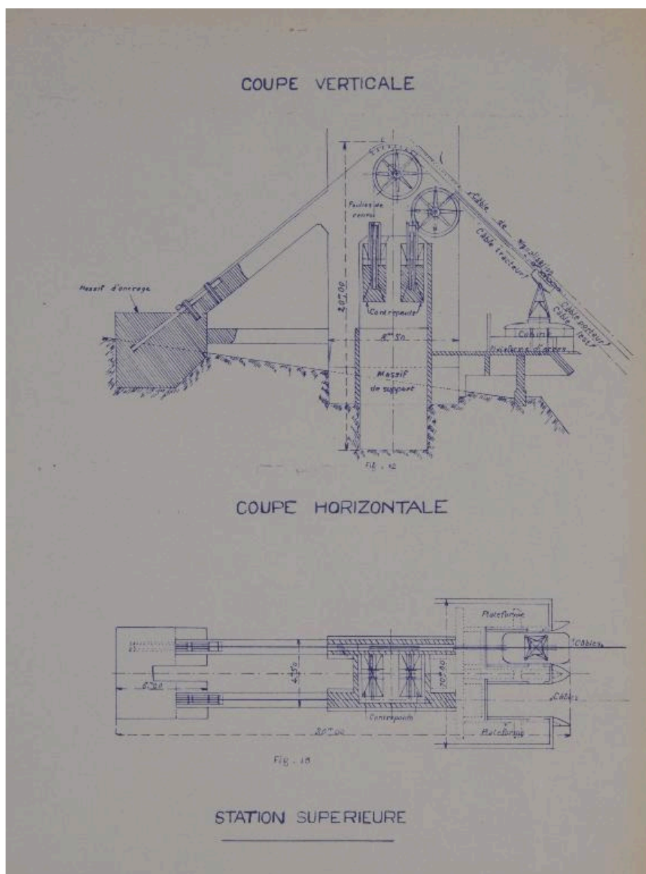
Gare supérieure : coupes verticale et horizontale
