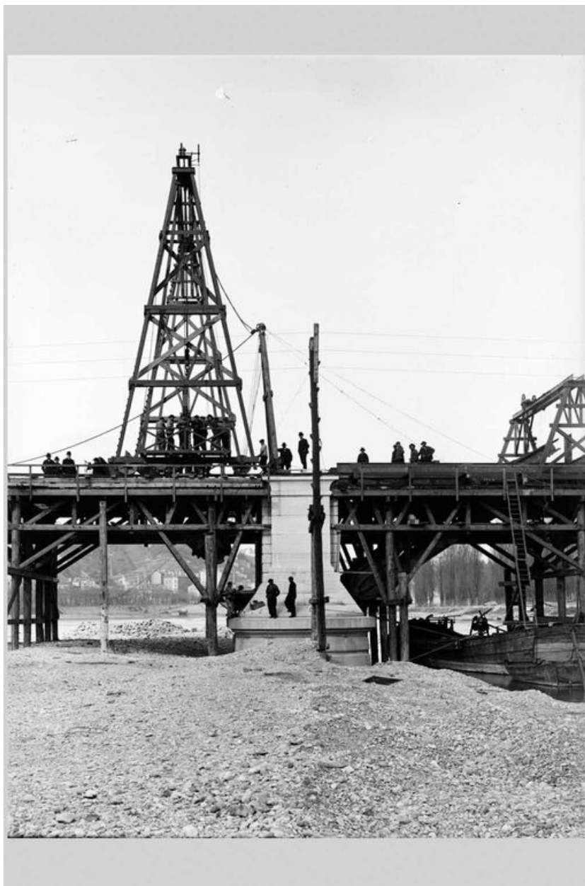
La construction du pont de la Boucle. La pile reposant sur l'îlot central du Rhône. Photographie, [1903] (Arch. mun. Lyon. 15 Ph 1815)
