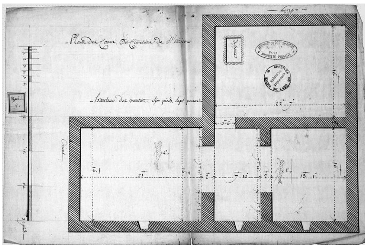
Plans des caves du cimetière de St-Nizier, par Charles-Antoine Roche et Cire Decrénice, 1777-1778
