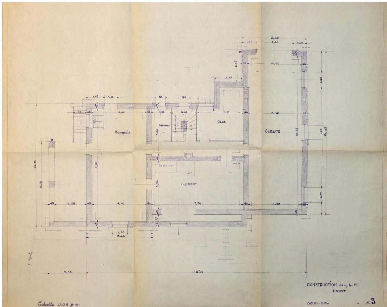
Royat, la maison M., plan du sous-sol semi-enterré, octobre 1950, Georges Guignabert architecte (Archives départementales du Puy-de-Dôme, Fonds de la Direction départementale de l'Équipement, 1611 W 47, PC n° 1822).
