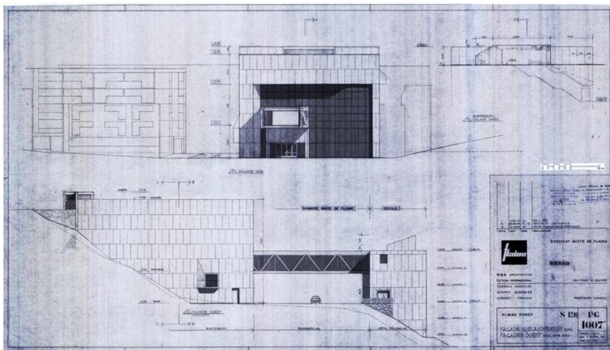
Elévation sud de l'auditorium. Elévation ouest de l'auditorium, de la passerelle et de l'hôtel. M.B. A architectes, 18 décembre 1984 (AC Arâches-la-Frasse)
