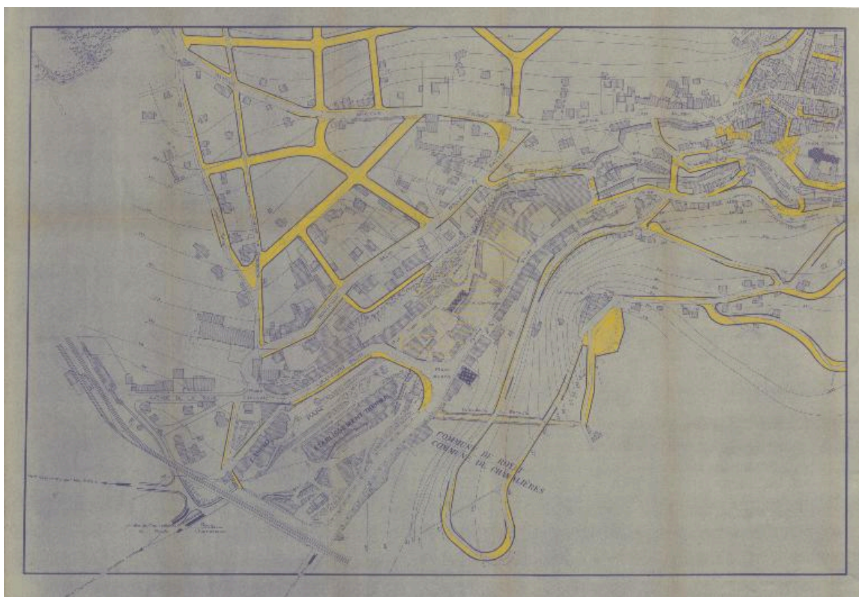
PAE de Royat (Puy-de-Dôme), 2e feuille sur 3, 1931
