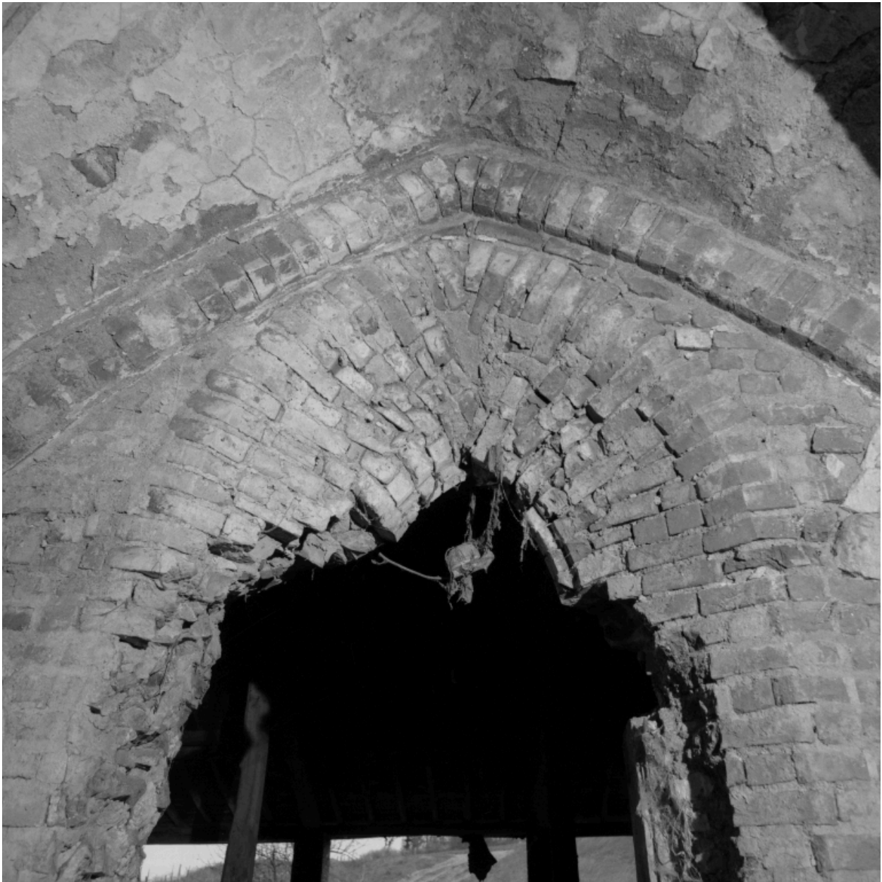
Détail de mise en oeuvre des briques dans une baie haute du bas côté nord, parement intérieur.
