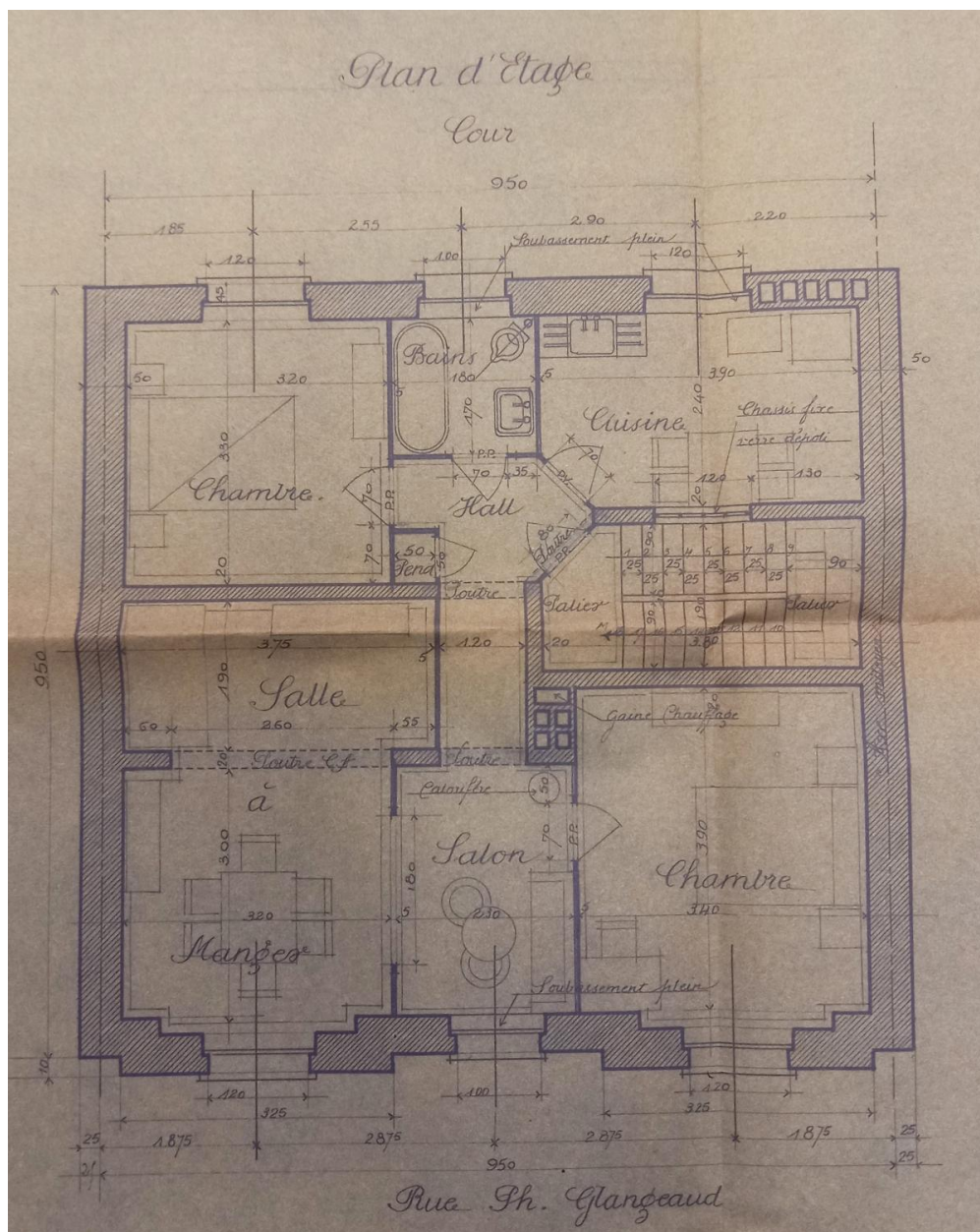
Plan des étages
