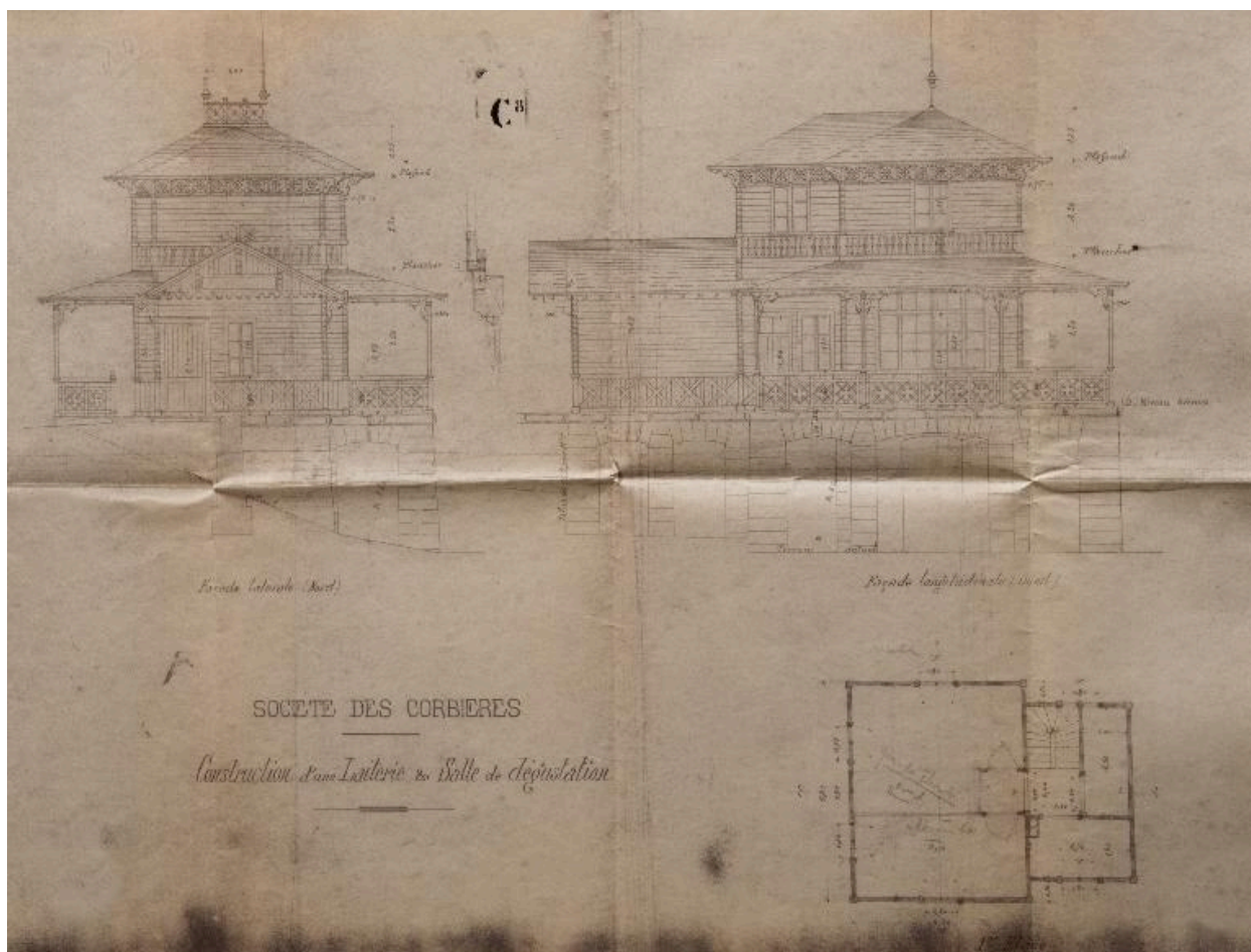
Laiterie : façades nord et ouest, plan du 1er étage, 1893
