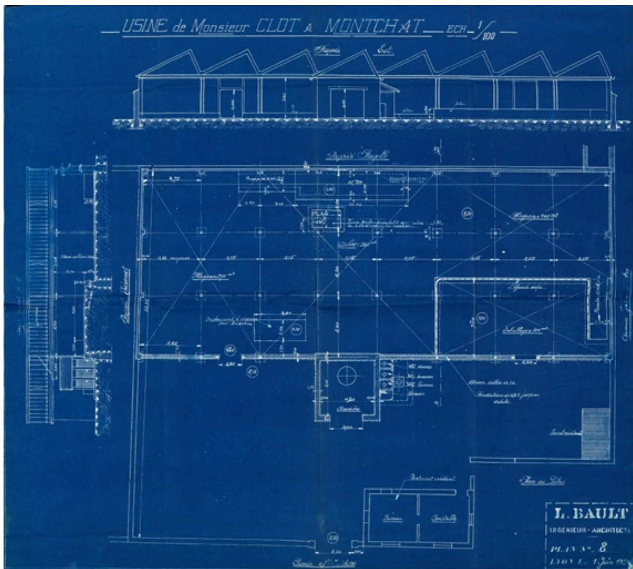
AC Lyon : 344 WP 096 PCA n°0348, plan, coupe élévation de l'usine de M. Clot par M. Bault, 1921
