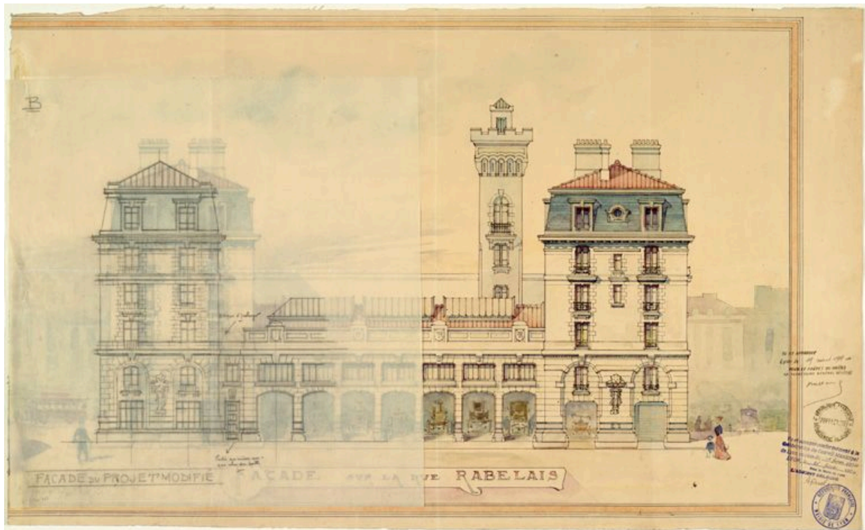
Elévation sur la rue Rabelais, avec la deuxième retombe
